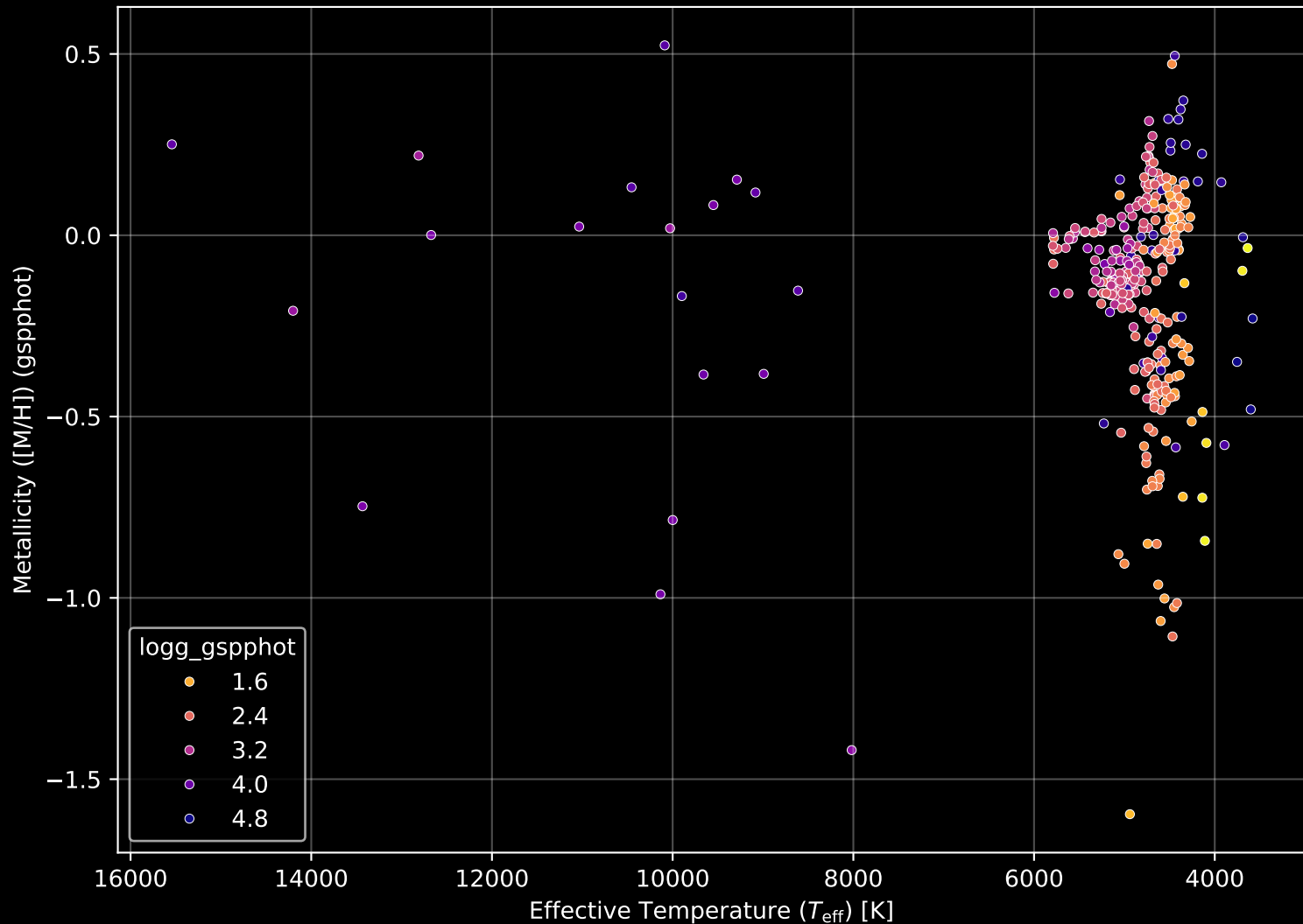
APOGEE DR17 Field: [120-12] Stellar Population Parameters (n= 370)
